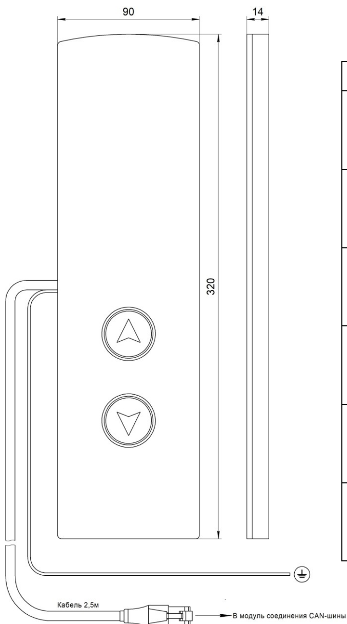
Рис.1 Внешний вид Вызывной пост ТОПАЗ (жгут RJ45) НШЕК.468381.210
